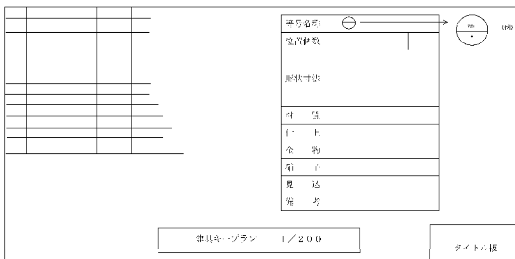
図－7 建 具 表
